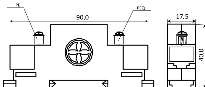
Рисунок 3. Габаритные размеры устройства Commeng FEP
