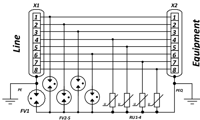
Рисунок 2. Функциональная схема устройства Commeng FEP
