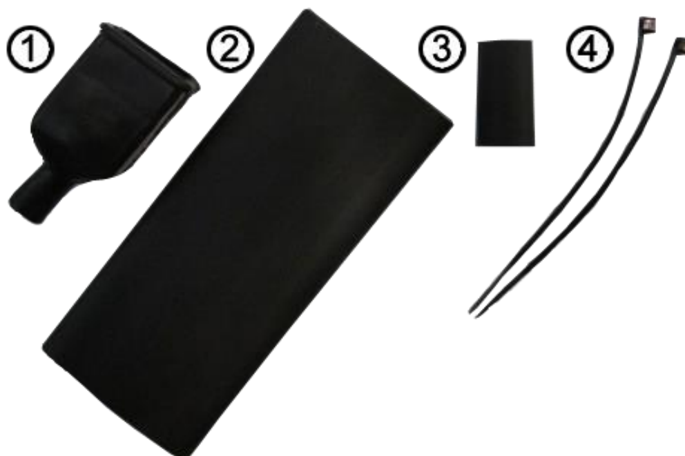
Рисунок 2. Монтажный комплект КМЕ-1
