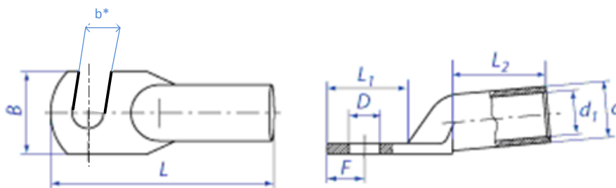
Рисунок 2. Основные габаритные размеры крюкового наконечника ТМЛ
