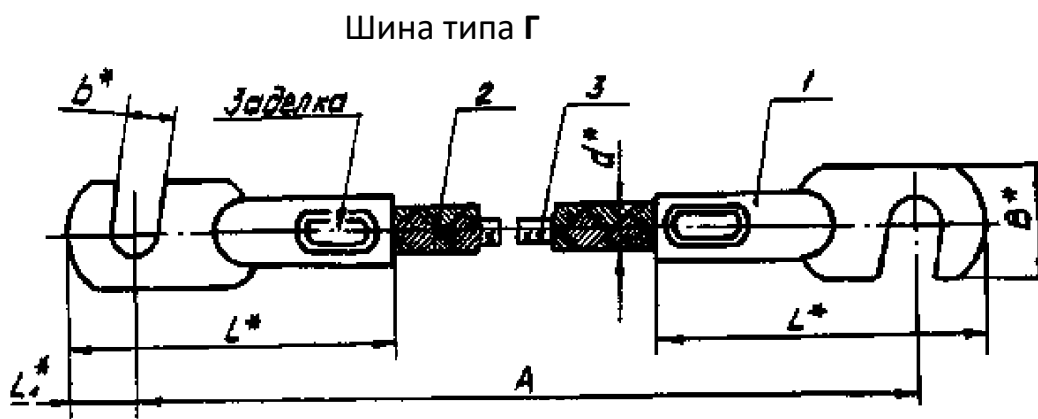
Рисунок 1. Габаритные размеры шины тип Г (1-наконечник; 2-плетёнка; 3 – провод)
